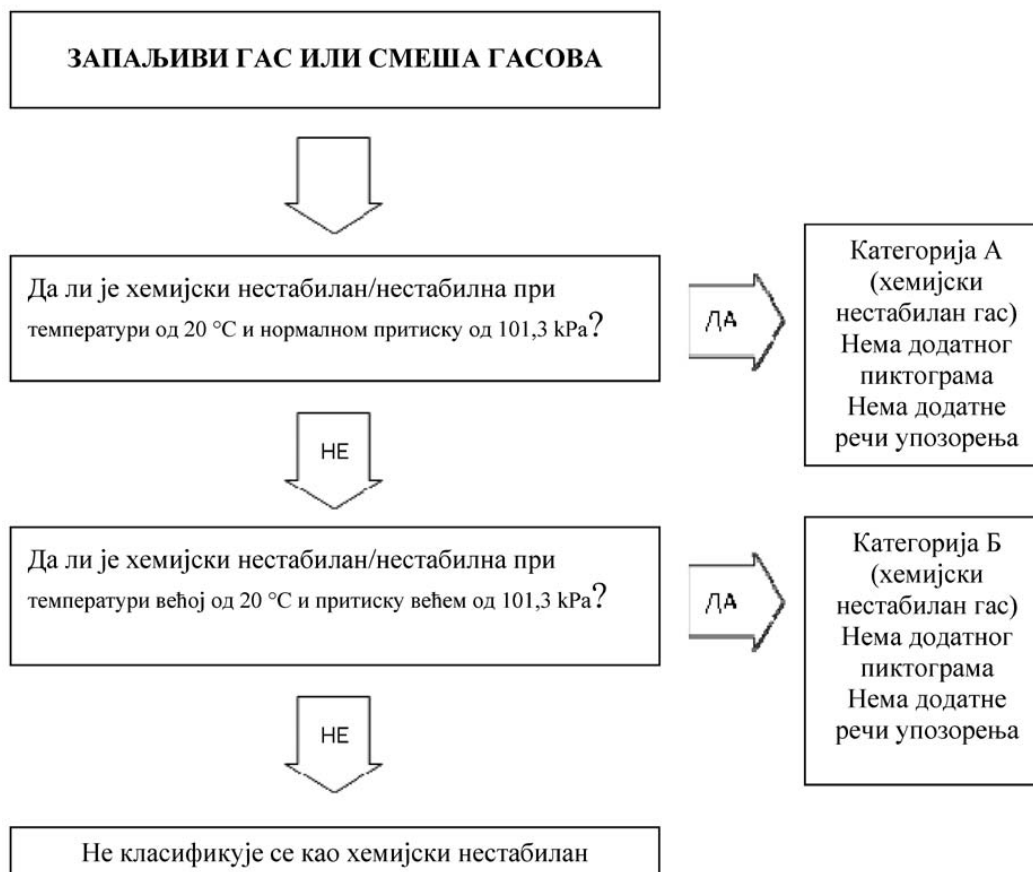
Слика 2.2.2. Поступак класификације хемијски нестабилних гасова
