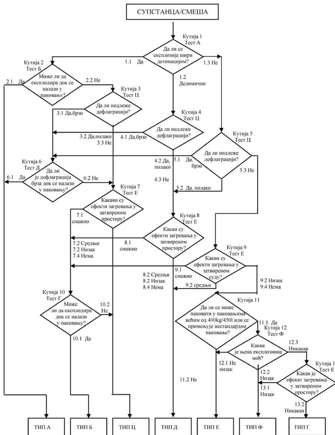
Слика 2.8.1. Самореактивне супстанце и смеше
