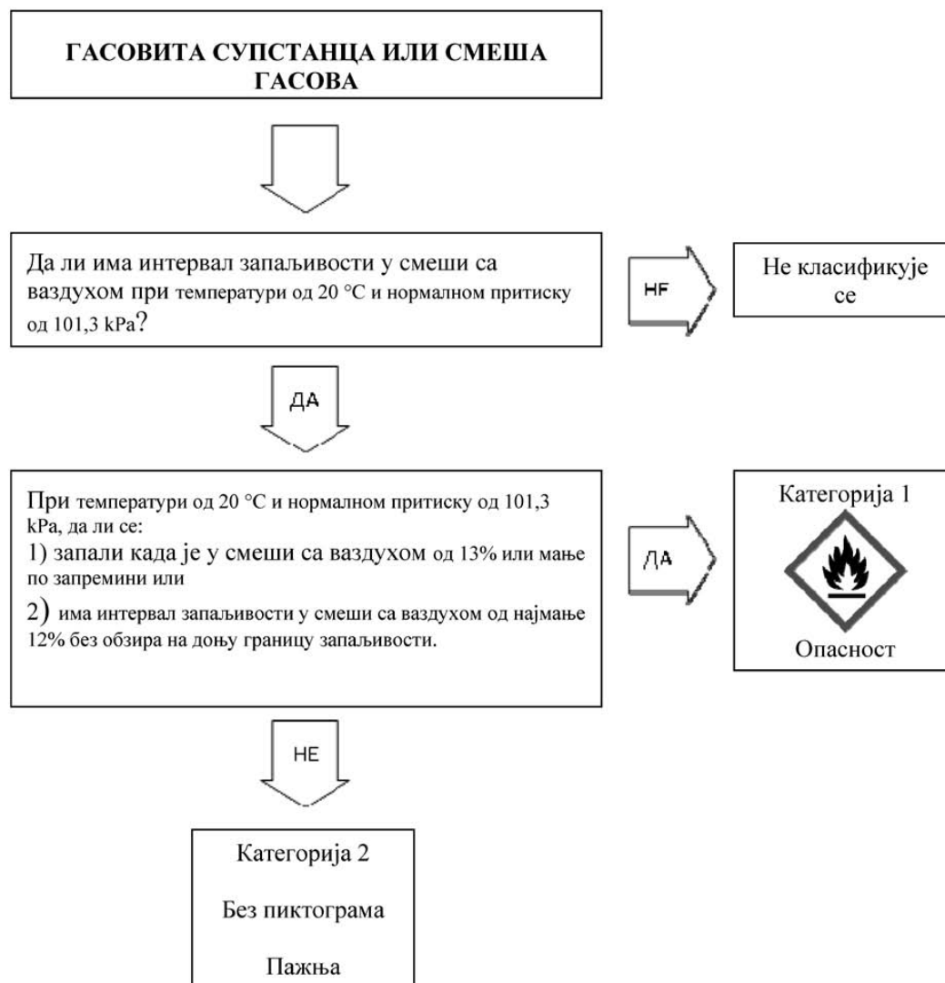
Слика 2.2.1. Поступак класификације запаљивих гасова
