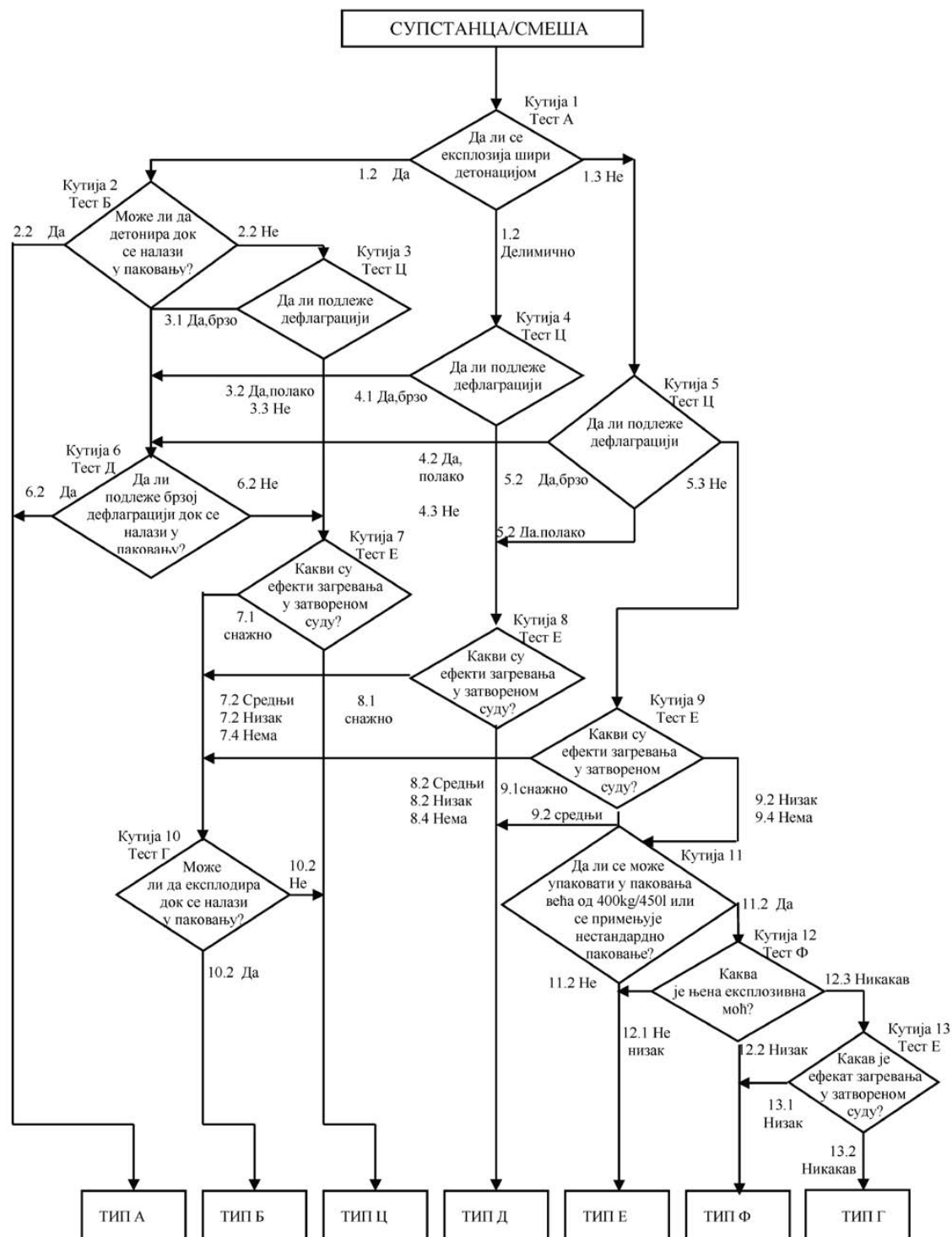
Слика 2.15.1. Органски пероксиди
